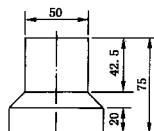
c) 加压块
