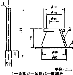
图 B1 试模及捣棒
