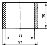
a) 圆筒
